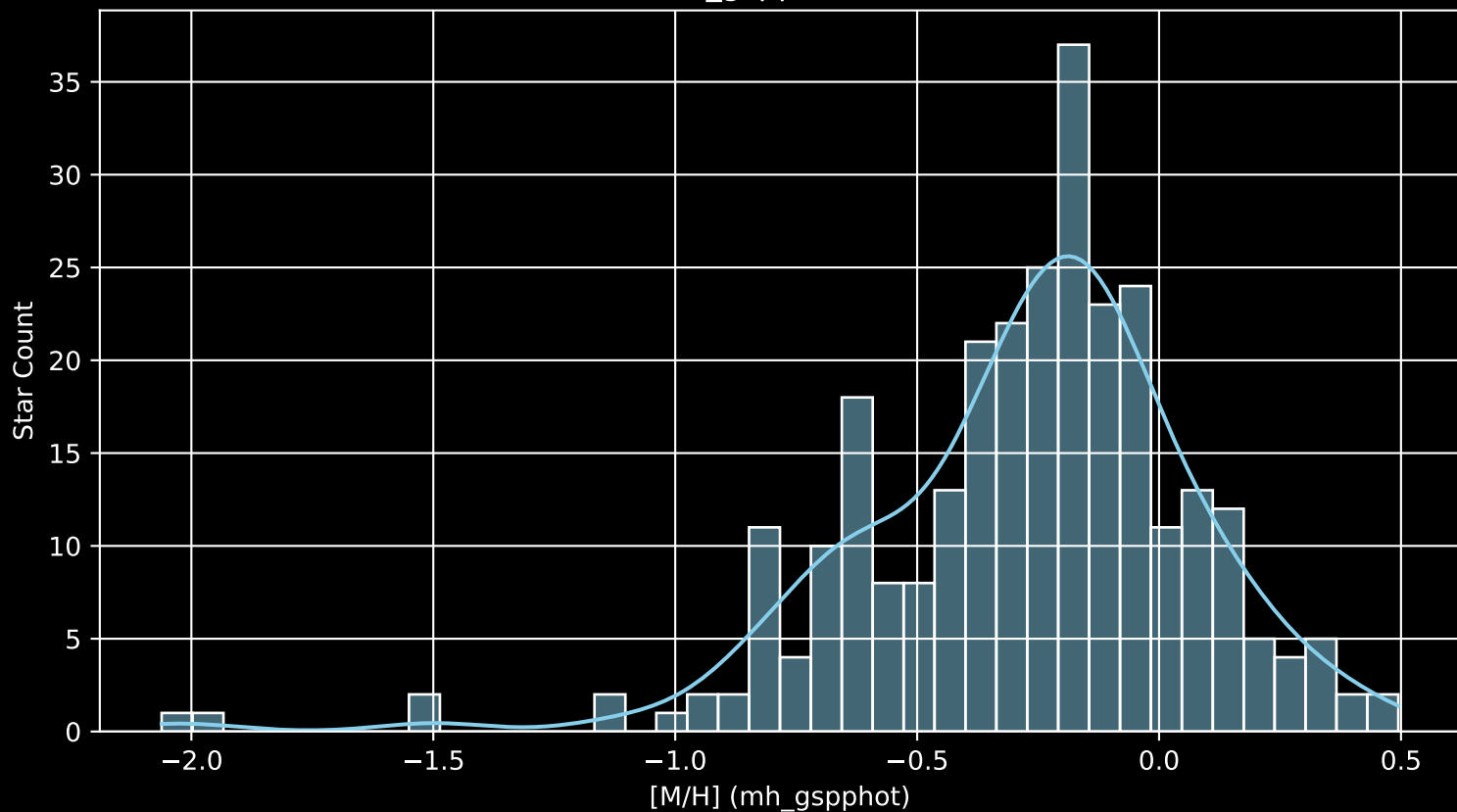
GALAH DR4 Field: [7013] [M/H] (mh_gspphot) (n= 289)
