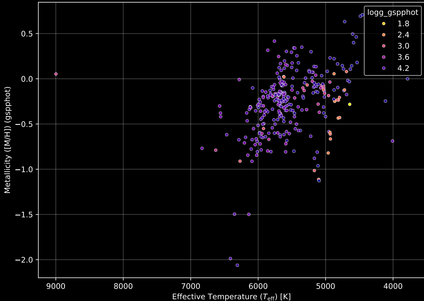
GALAH DR4 Field: [7013] Stellar Population Parameters (n= 292)
